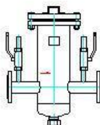
ФГ-ГК-50-01-Ф, ФГ-ГК-50-У-03-Ф, ФГ-ГК-80-03-Ф, ФГ-ГК-100-03-Ф
