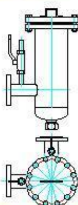
ФГ-ГК-50-У-05-Ф, ФГ-ГК-80-05-Ф, ФГ-ГК-100-05-Ф
