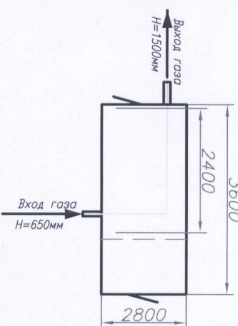
План входа и выхода газа в ГРПБ
